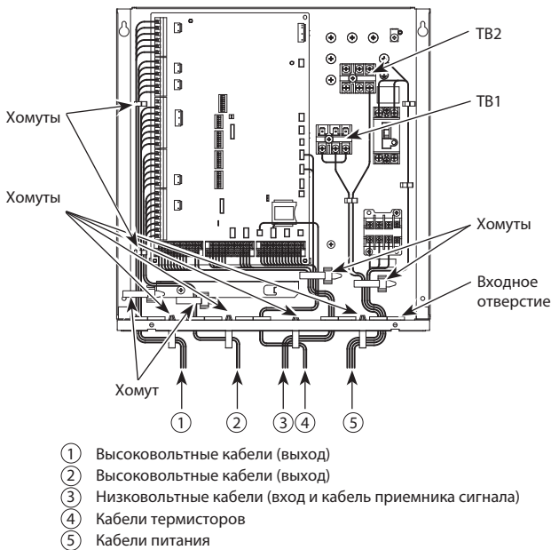
Рис. 4.1.1 Проводка PAC-IF062/063B-E
