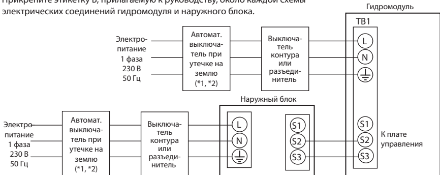
Рис. 3.2.17 Электрические соединения, 1 фаза
