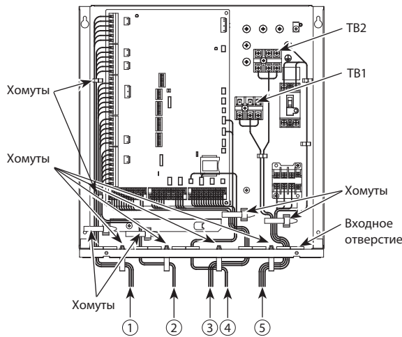
Рис. 4.1.4 Проводка PAC-IF062/063B-E
