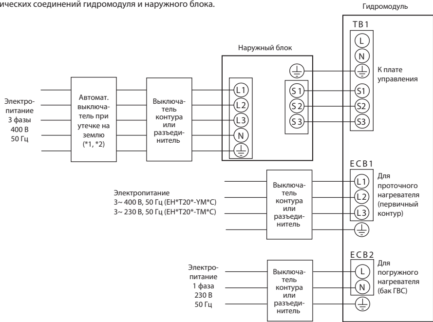
Рис. 3.1.4 Электрические соединения, 3 фазы
