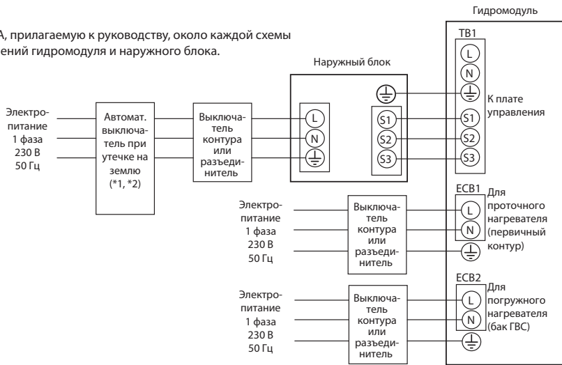
Рис. 3.1.3 Электрические соединения, 1 фаза
