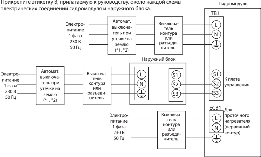
Рис. 3.2.12 Электрические соединения, 1 фаза
