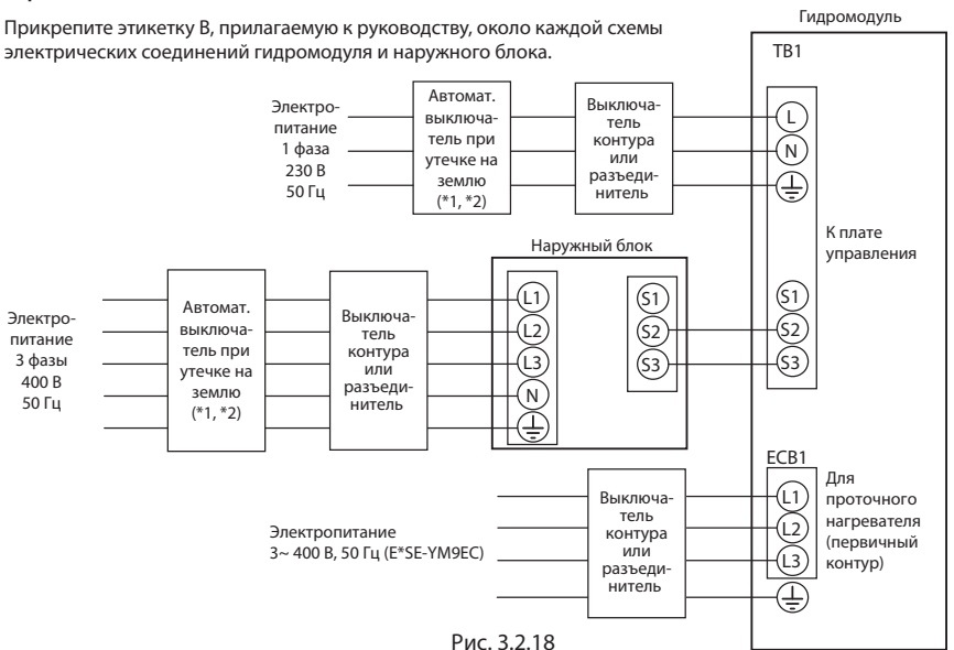
Рис. 3.2.18 Электрические соединения, 3 фазы
