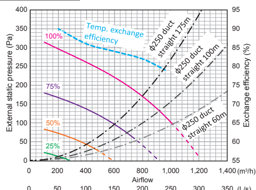
LGH-80RVS-E
